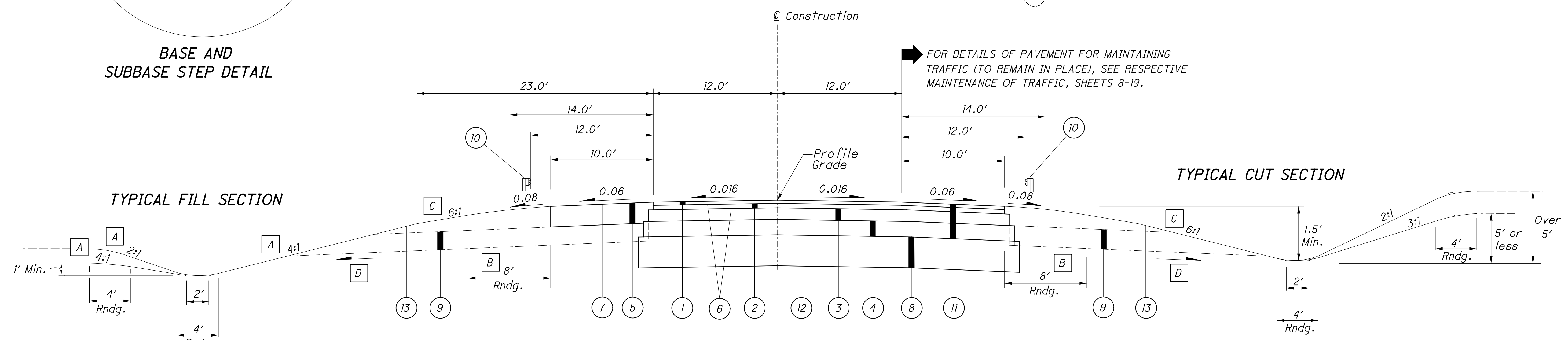
NORMAL SECTION - U.S. 46 Sta. 635+75.00 to Sta. 642+81.37 Sta. 638+22.44 to Sta. 640+48.86
